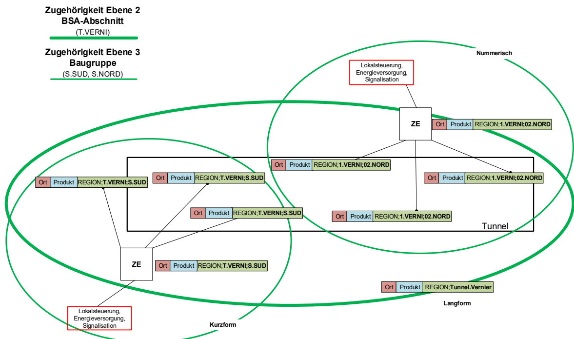
Abb. 6.2 Zugehörigkeitsbezogene Struktur für die Gliederungsebenen 2 „BSA-Abschnitt“ und 3 „Baugruppe“.
