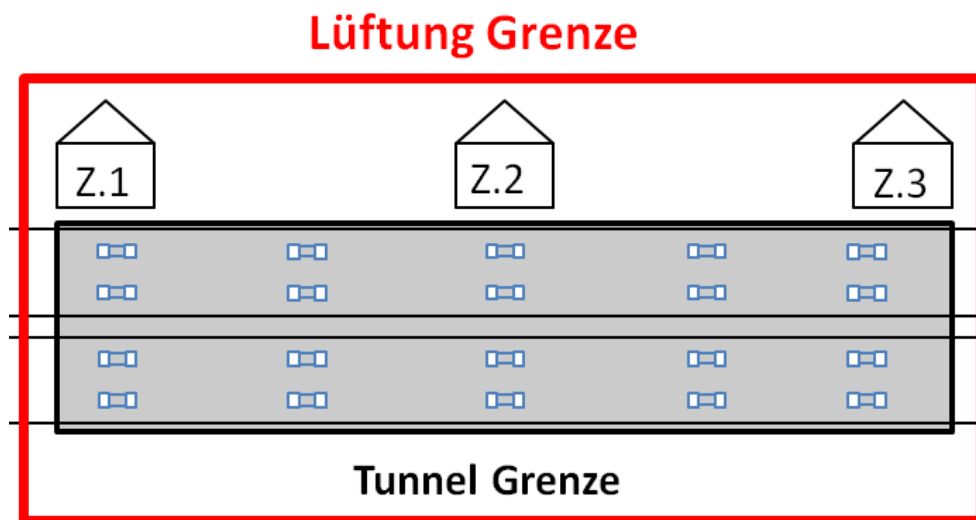
Abb. 5.8 Schematische Darstellung des Tunnels Grenze. Im Tunnel Grenze gibt es je Fahrrichtung 10 Strahlventilatoren, welche die Lüftung im Tunnel gewährleisten.
