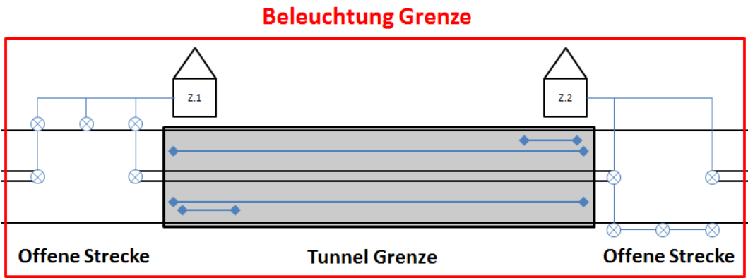
Abb. 5.6 Schematische Darstellung des Tunnel Grenze mit Vorzonenbeleuchtung auf der angrenzenden offenen Strecke.
