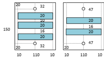
Abbildung 4-144: Masse für Tafeltyp «Standortfeld»
