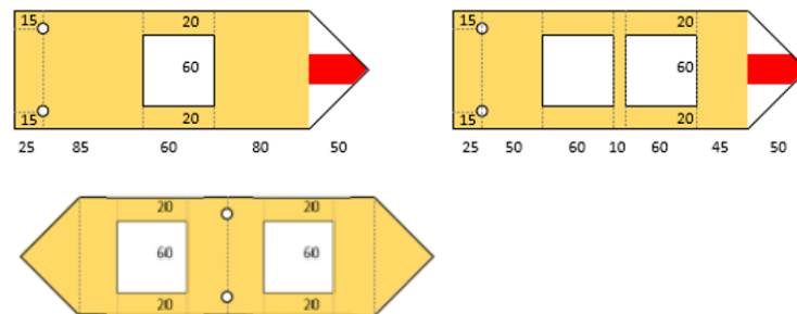
Abbildung 4-143: Masse für Tafeltyp «Richtungszeiger mit quadratischen Symbolen»
