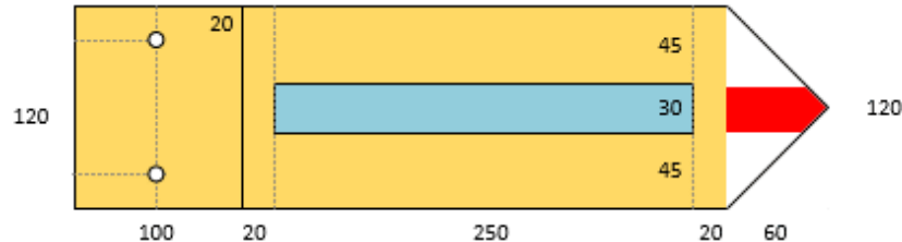
Abbildung 4-140: Masse für Tafeltyp «Zielwegweiser»
