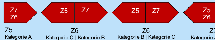
Abbildung 4-65: RSL: Signalisation unterschiedlicher Standortkategorien pro Richtung
