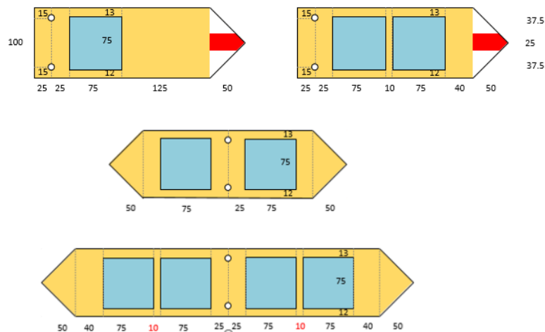
Abbildung 4-142: Masse für Tafeltyp «Richtungszeiger mit Routenfelder»
