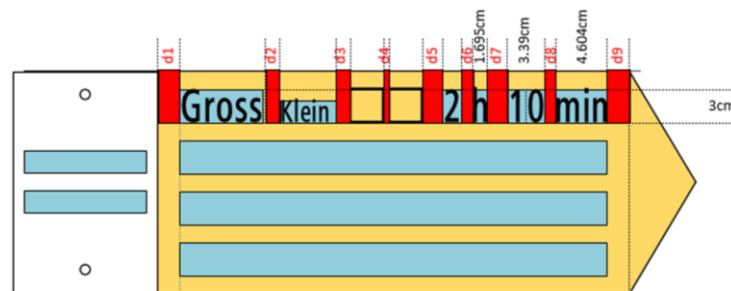
Abbildung 4-134: Abstände für Tafeltyp «Wegweiser mit Ziel- und Zeitangaben»
