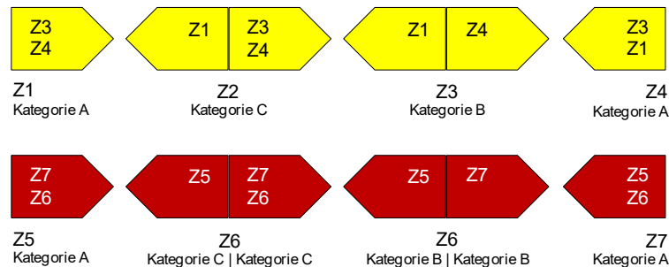
Abbildung 4-64: RSL: Signalisation der Standortkategorien A, B und C
