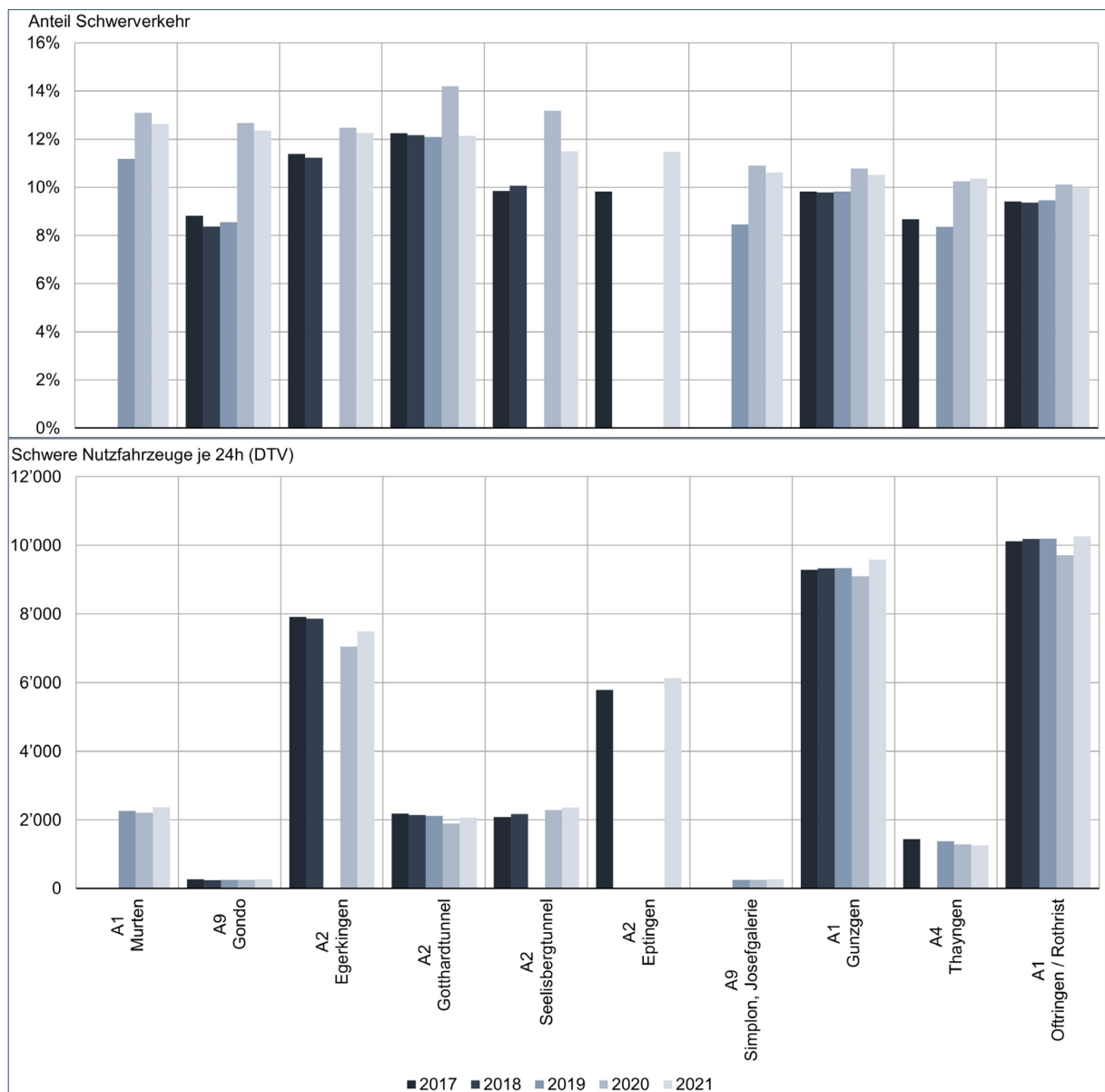
Abbildung 19: Schwerverkehrsbelastungen der zehn Querschnitte mit den höchsten Schwerverkehrsanteilen 2021 Quellen: ASTRA: SASVZ, ASTRA: VMON
