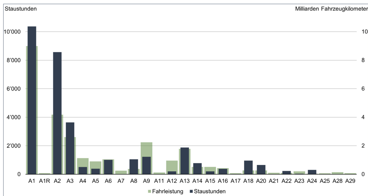
Abbildung 23: Stautunden 2021 nach Nationalstrassen (inkl. NEB) Quellen: ARE: VM-UVEK, ASTRA: SASVZ, ASTRA: VMON, Viasuisse
