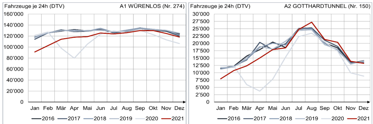
Abbildung 14: Typische Jahresganglinien DTV Quellen: ASTRA: SASVZ, ASTRA: VMON
