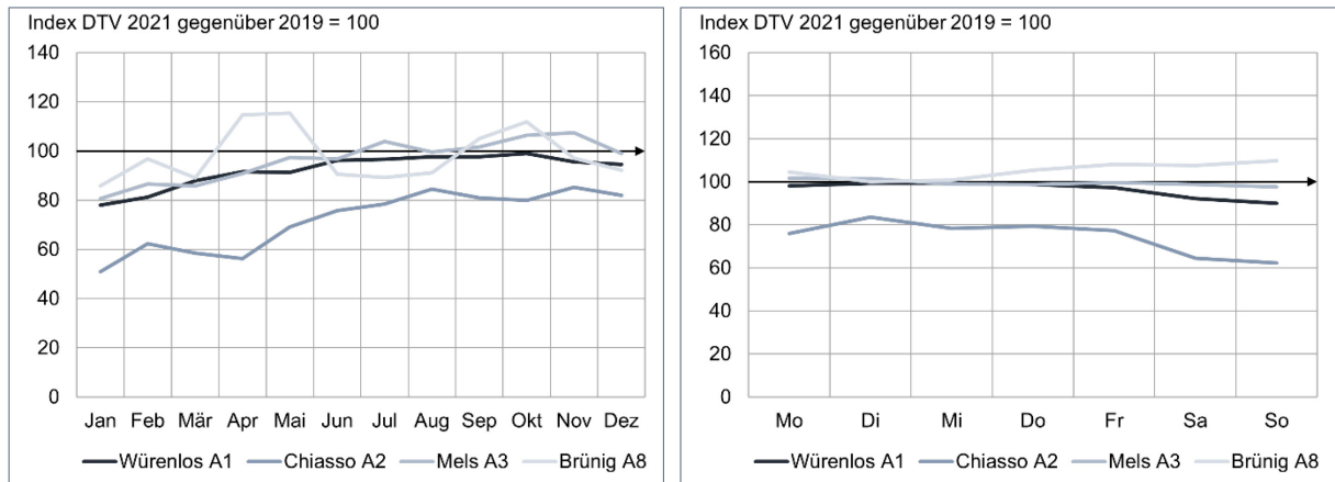
Abbildung 50: Jahresganglinien DTV (links) und Wochenganglinie (rechts) ausgewählte Querschnitte aus dem Jahr 2021 im Vergleich zu 2019
