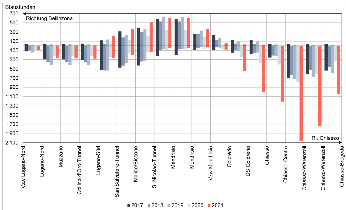
Abbildung 41: Entwicklung der Staustunden auf der A2 zwischen Lugano und Chiasso
