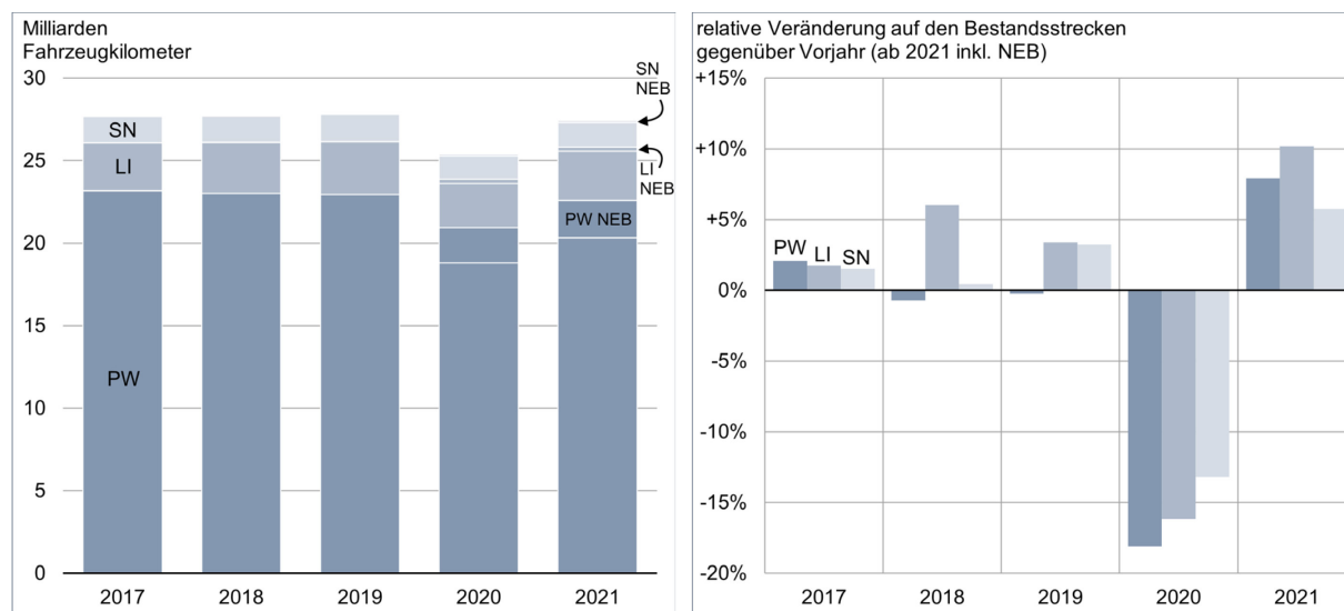
Abbildung 5: Verkehrsentwicklung auf dem Nationalstrassennetz nach Personen- und Güterverkehr
