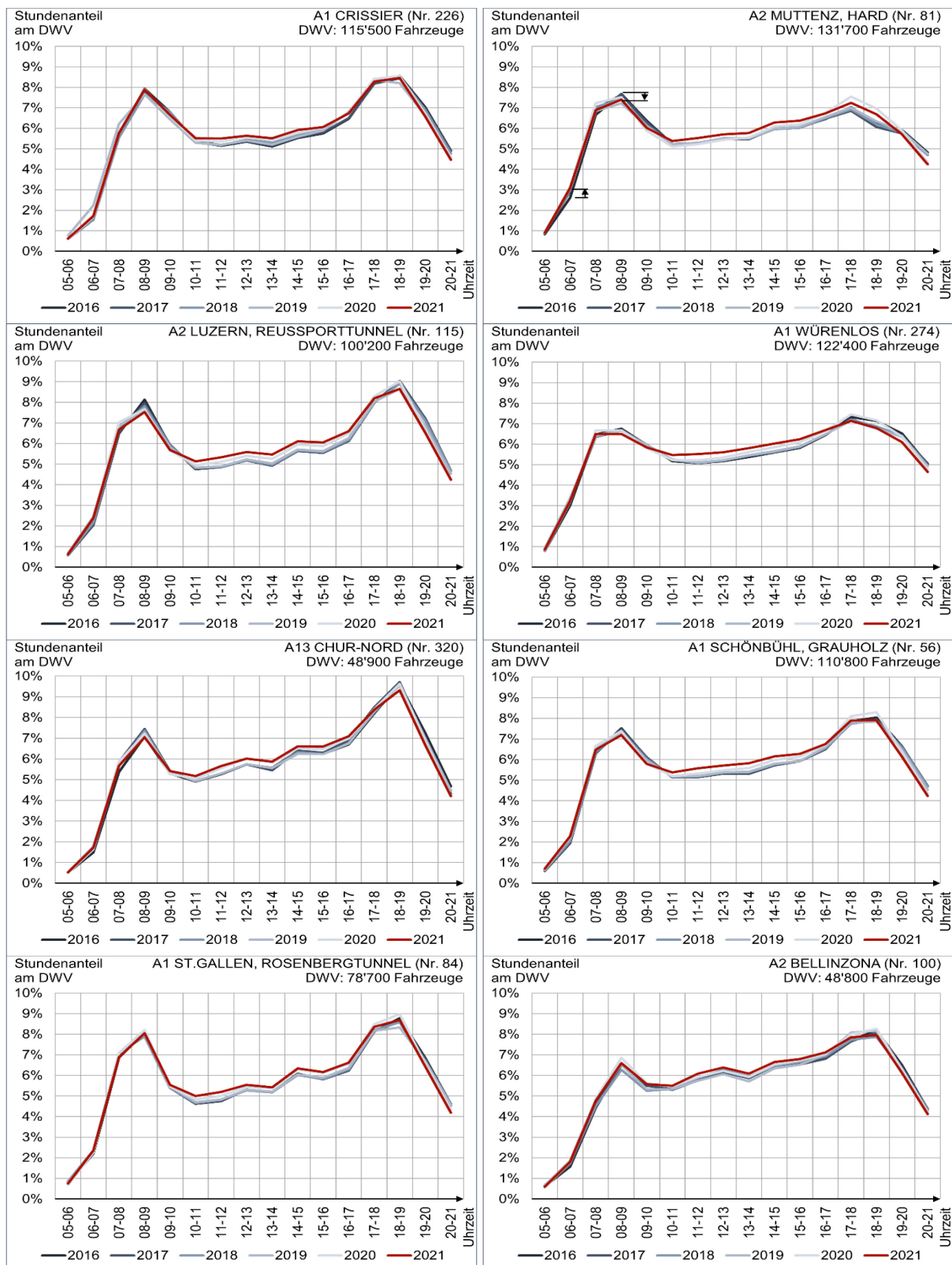
Abbildung 17: Tagesganglinien DWV an ausgewählten Zählstellen aus allen Landesteilen ↓↑ beispielhafte Kennzeichnung der retrospektiv beobachteten Spitzenstundenverschiebungen Quellen: ASTRA: SASVZ, ASTRA: VMON
