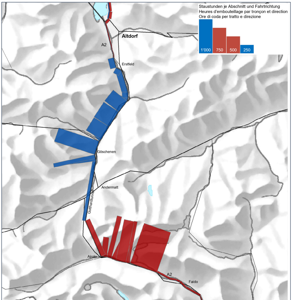
Abbildung 40: Stautunden 2021 auf den Nationalstrassen in der Region Gotthard Quellen: ASTRA: VMON, Viasuisse
