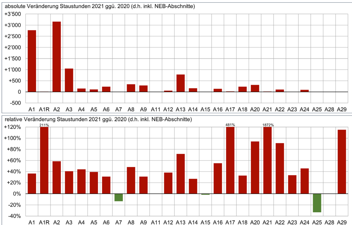
Abbildung 25: Veränderung der Stautunden 2021 gegenüber 2020 nach Nationalstrassen (inkl. NEB) Quellen: ASTRA: VMON, Viasuisse
