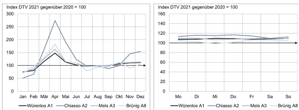
Abbildung 49: Jahresganglinien DTV (links) und Wochenganglinie (rechts) ausgewählte Querschnitte aus dem Jahr 2021 im Vergleich zu 2020
