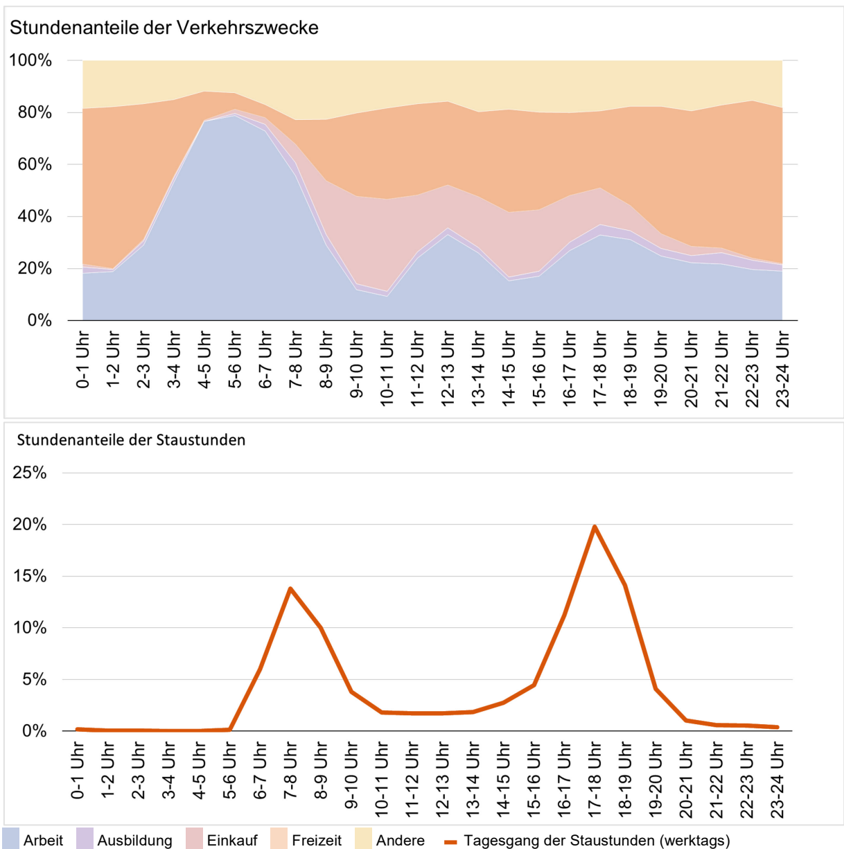
Abbildung 47: Stundenanteile der Verkehrszwecke 2015 und der Stautunden 2019 für Werktage Quelle: Viasuisse 2019, Mikrozensus Mobilität und Verkehr 2015, Eigene Darstellung
