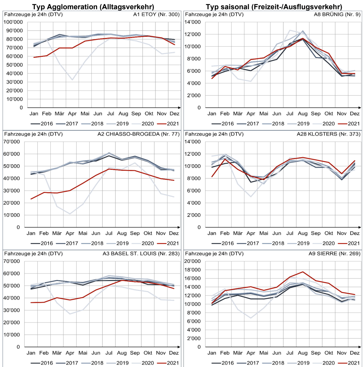
Abbildung 15: Ausgewählte Jahresganglinien DTV im Corona-Jahr 2020 für das Jahr 2021 Quellen: ASTRA: SASVZ, ASTRA: VMON
