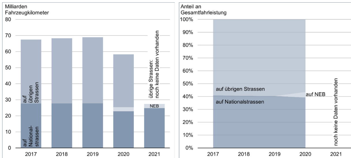
Abbildung 2: Entwicklung des Gesamtverkehrs (Personen und Güter) auf dem gesamten Strassennetz Quellen: ARE: VM-UVEK, ASTRA: SASVZ, ASTRA: VMON, BFS: PV-L 3
