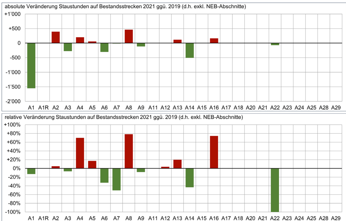
Abbildung 26: Veränderung der Stautunden 2021 gegenüber 2019 nach Nationalstrassen (exkl. NEB) Quellen: ASTRA: VMON, Viasuisse
