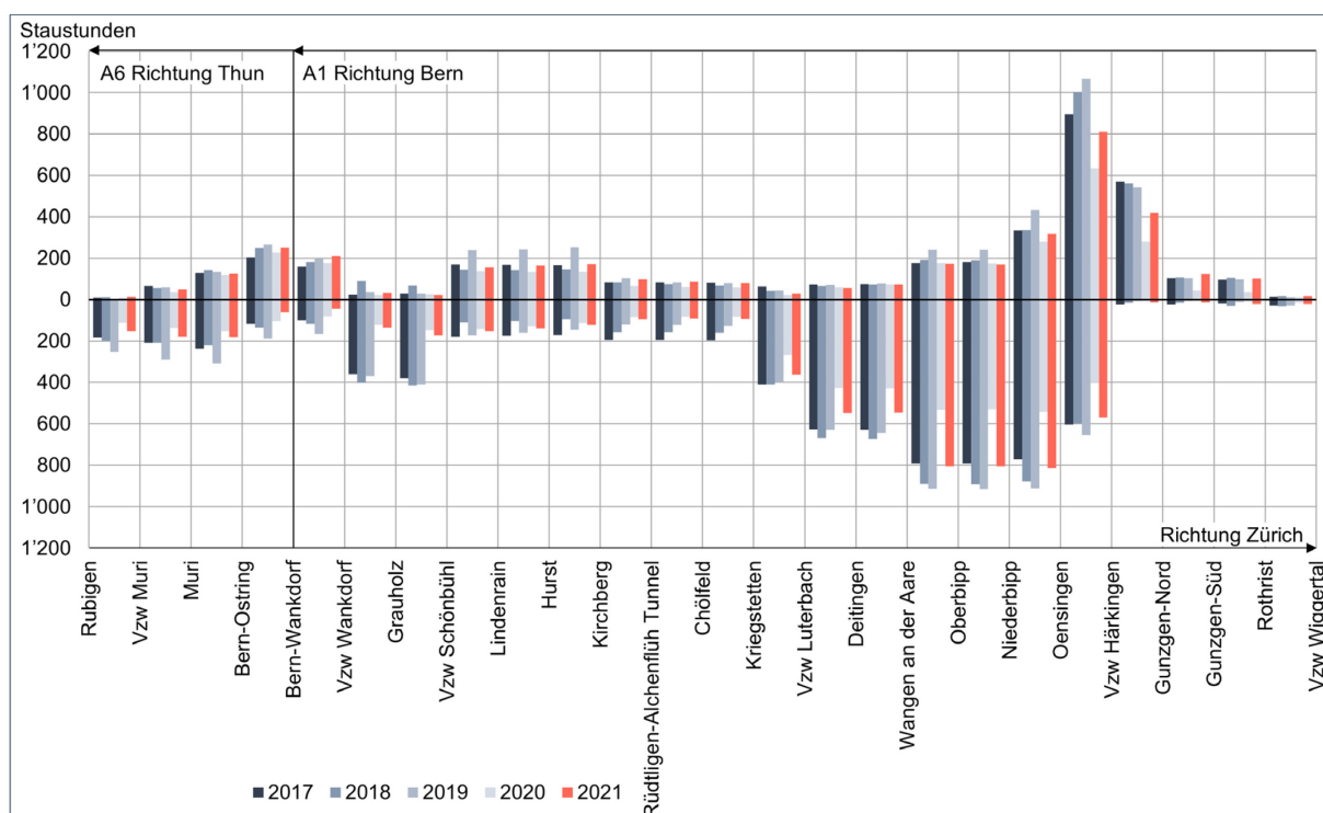
Abbildung 34: Entwicklung der Stautunden auf A6 und A1 zwischen Rubigen und Wiggertal Quellen: ASTRA: VMON, Viasuisse
