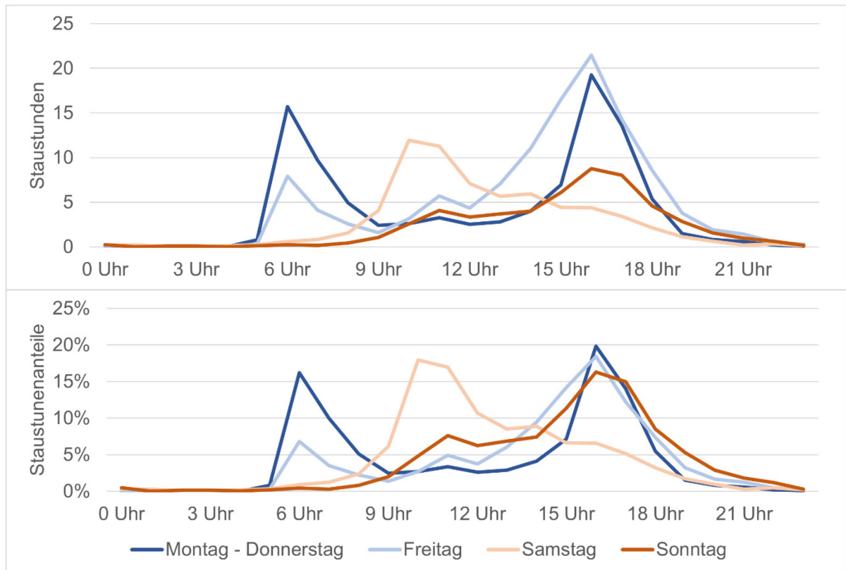
Abbildung 46: Stautunden und Stautundenanteile 2021 auf den Nationalstrassen im Tagesgang nach Tagestyp Quellen: ASTRA: VMON, Viasuisse, Eigene Darstellung
