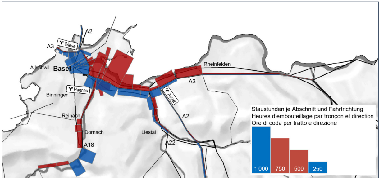
Abbildung 30: Stautunden 2021 auf den Nationalstrassen in der Region Basel
