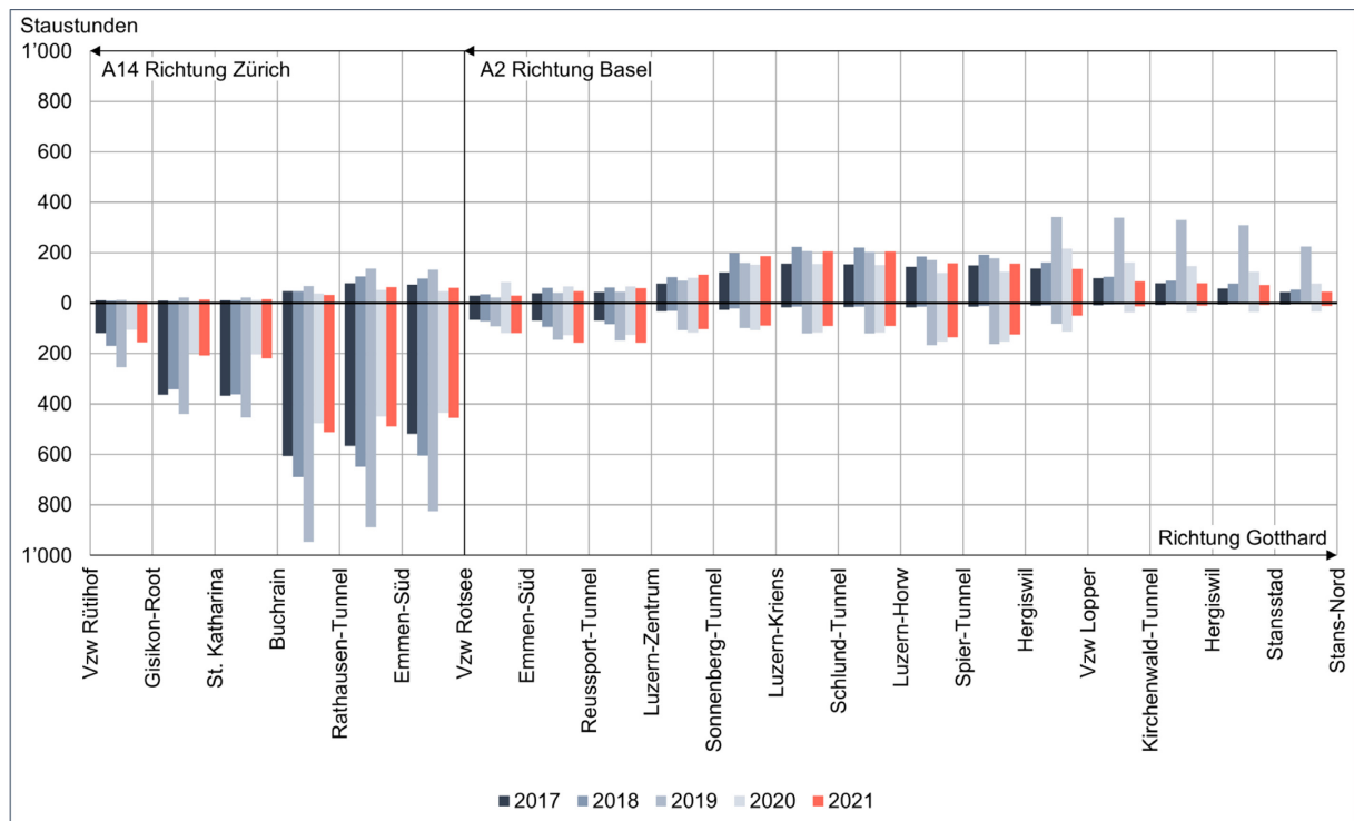
Abbildung 33: Entwicklung der Stautunden auf A14 und A2 zwischen Rütihof und Stans Quellen: ASTRA: VMON, Viasuisse
