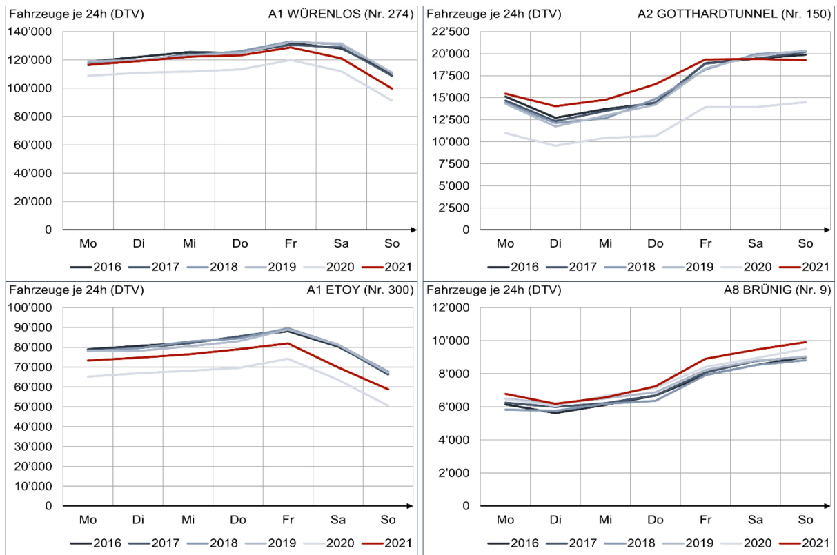
Abbildung 16: Typische Wochenganglinien DTV Quellen: ASTRA: SASVZ, ASTRA: VMON
