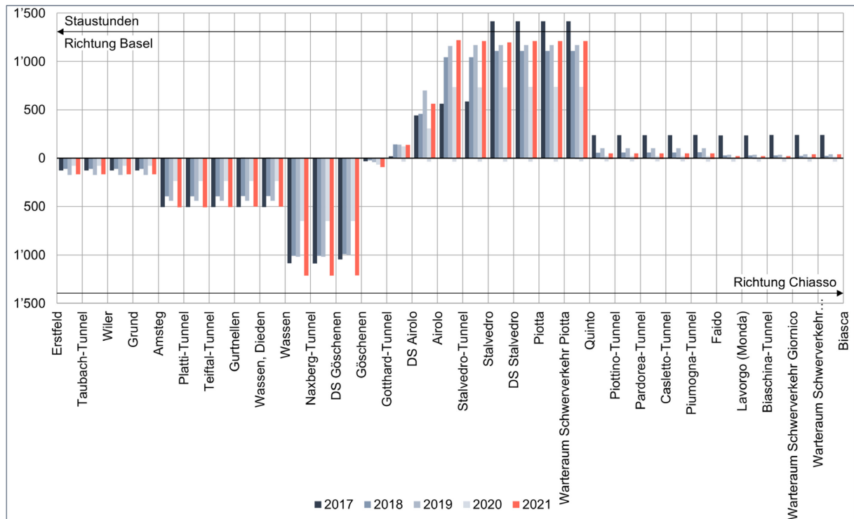
Abbildung 39: Entwicklung der Stautunden auf der A2 zwischen Erstfeld und Biasca Quellen: ASTRA: VMON, Viasuisse
