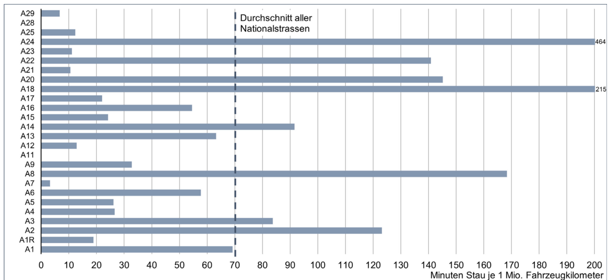
Abbildung 24: Fahrleistungsbezogene Stauintensität 2021 nach Nationalstrassen (inkl. NEB-Strecken)
