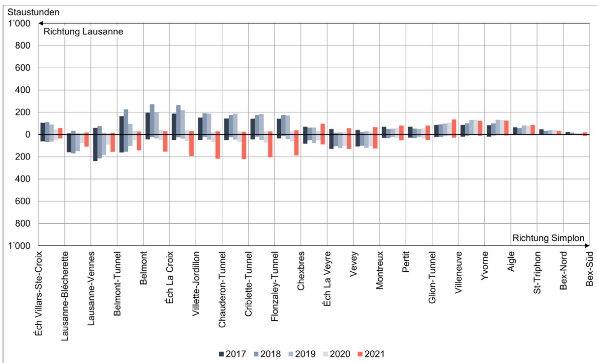
Abbildung 38: Entwicklung der Stautunden auf der A9 zwischen Villars-Ste-Croix und Bex Quellen: ASTRA: VMON, Viasuisse
