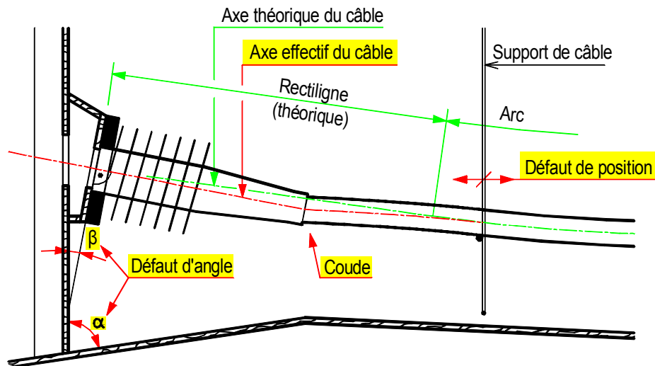
Fig. II.6 Conditions géométriques.
