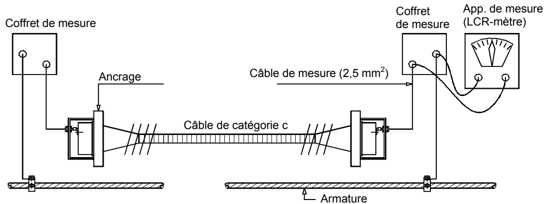
Fig. I.2 Disposition des installations pour la mesure de la résistance en cas de raccordement aux deux extrémités du câble de précontrainte.
