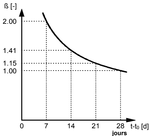
Fig. I.6 Facteur de conversion \beta permettant de tenir compte de l'incidence du temps sur la résistance électrique mesurée.
