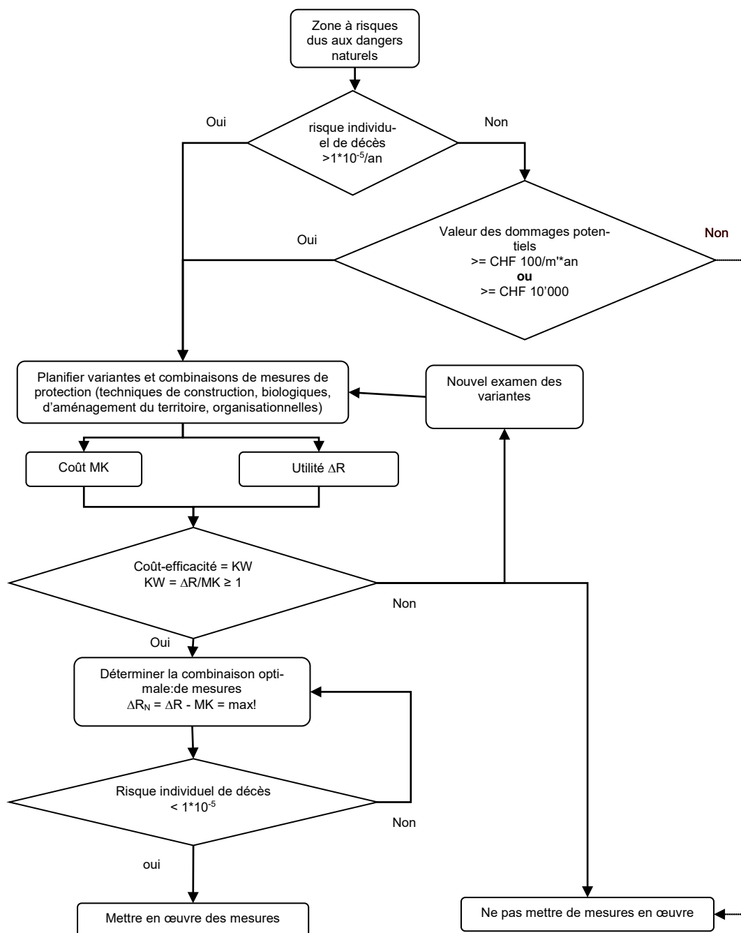
Fig. 7.3 Procédé d'appréciation des risques et de définition des priorités pour la planification de mesures contre les risques individuels liés aux personnes.
