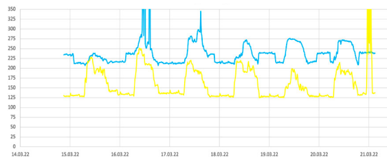
Bözberg Consommation électrique en kW
